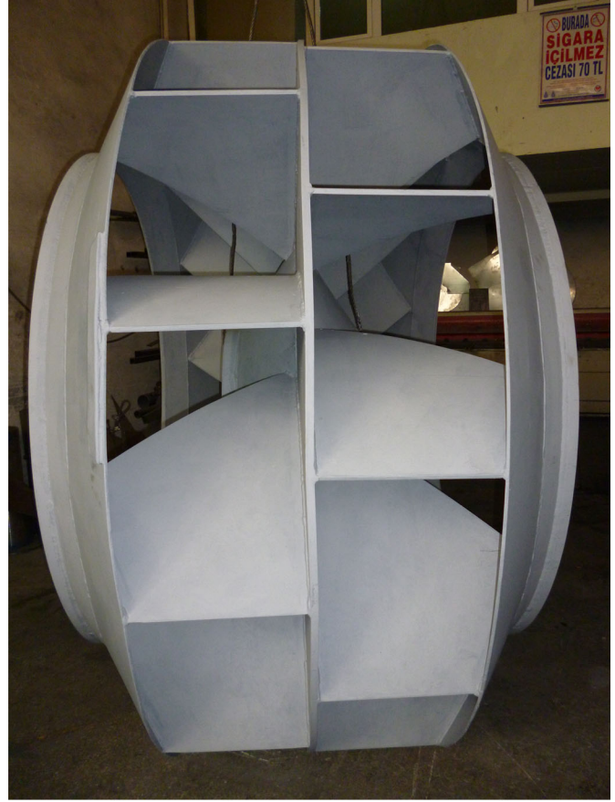
HÜCRELİ FAN PERVANESİ
